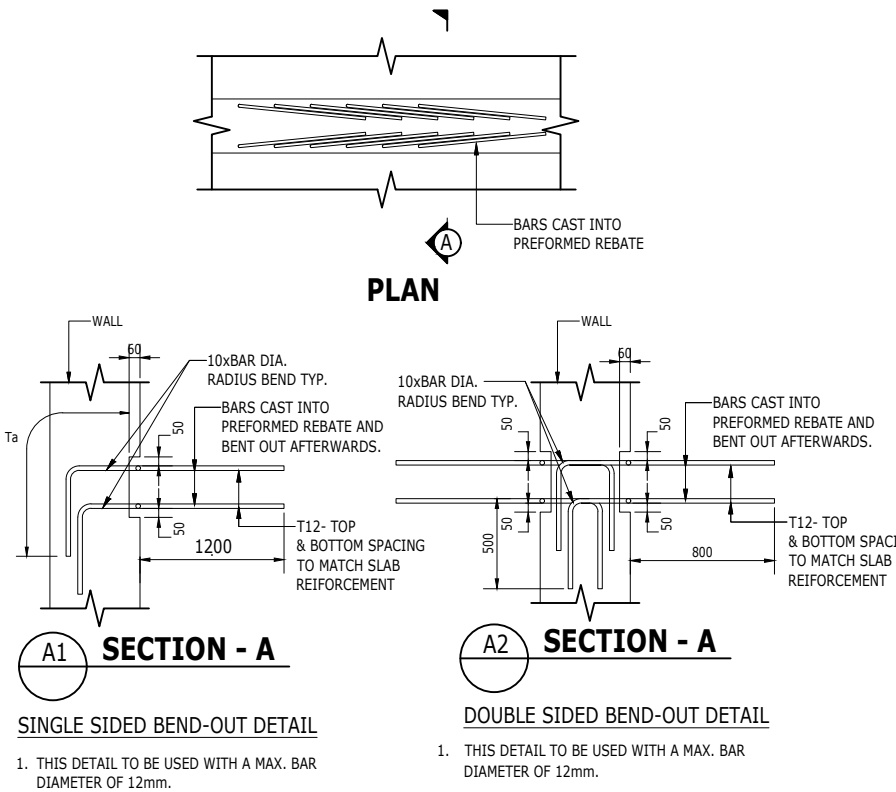
7 BEND-OUT DETAIL SCALE: N.T.S.
