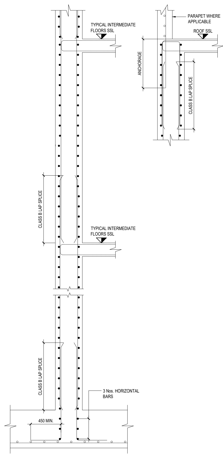
8 TYPICAL SHEAR WALL SECTION SCALE: N.T.S.
