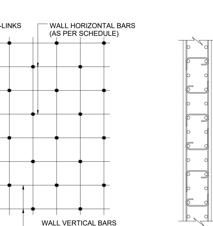
8 TYPICAL SHEAR WALL SECTION SCALE: N.T.S.
